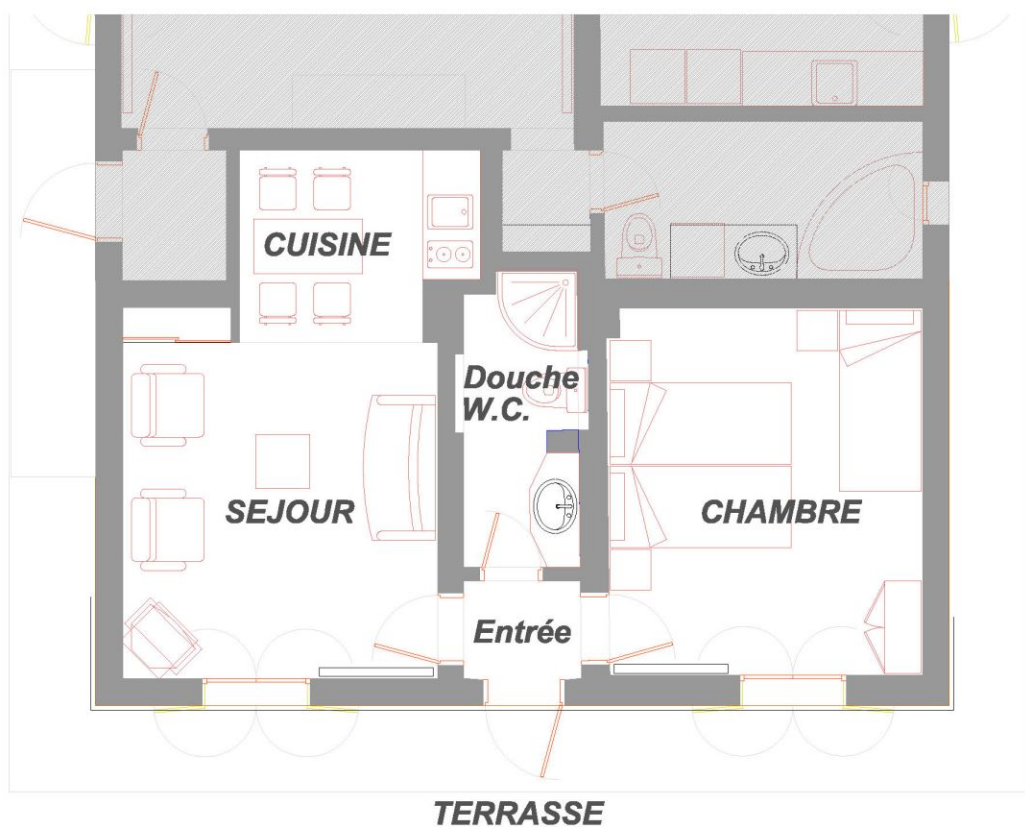
APPARTEMENT 2 échelle 1:50e
